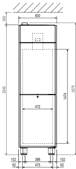
Front aanzicht
